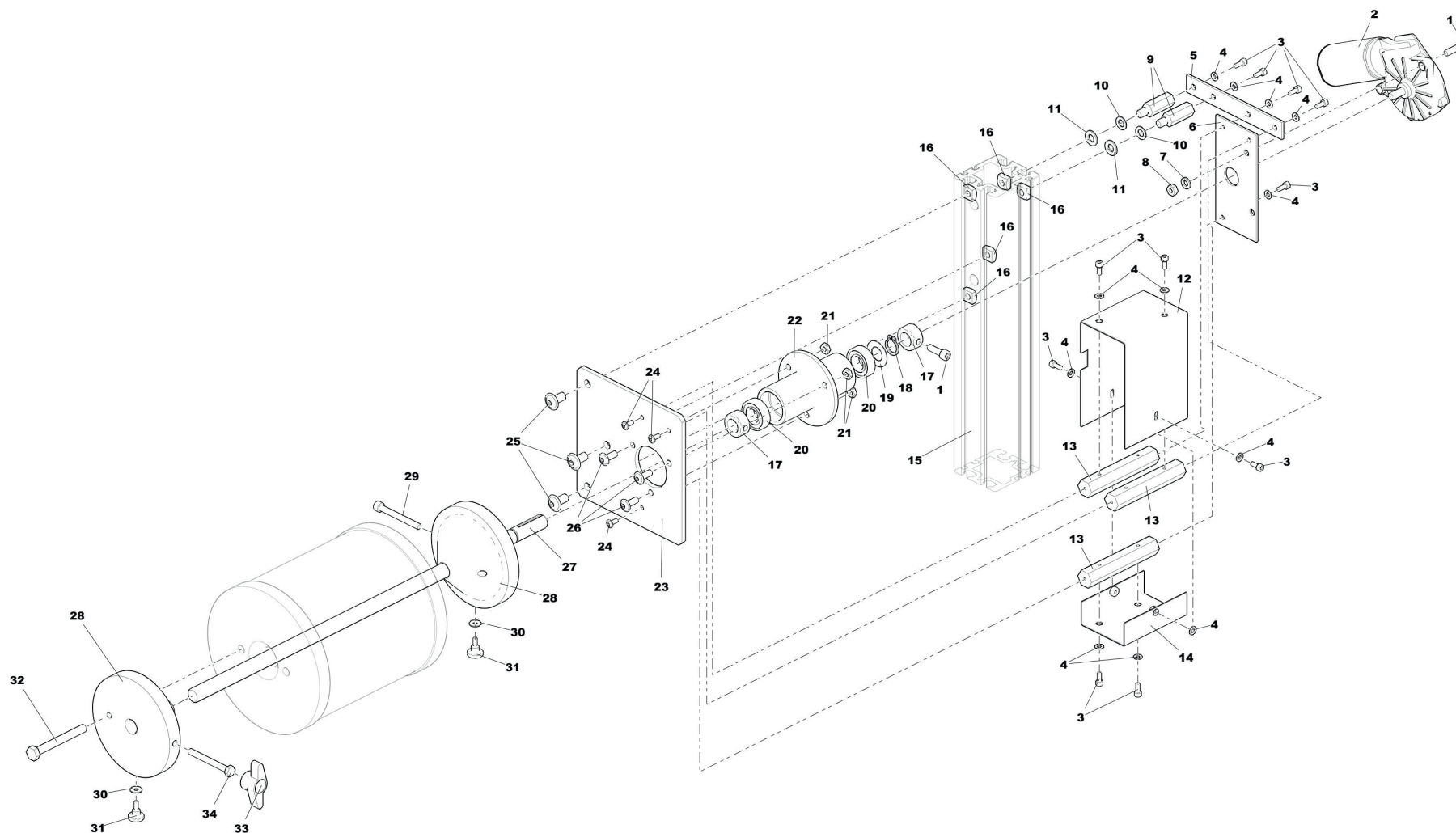
DLE-310_031_908_(H)-Spulenaufnahme & Antrieb
