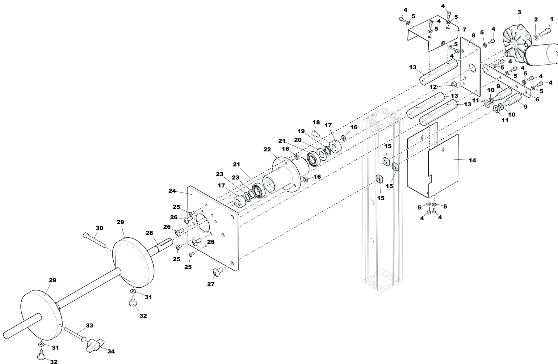
TDLE - 310 031 929 - Spulenaufnahme lks. m. Antrieb
