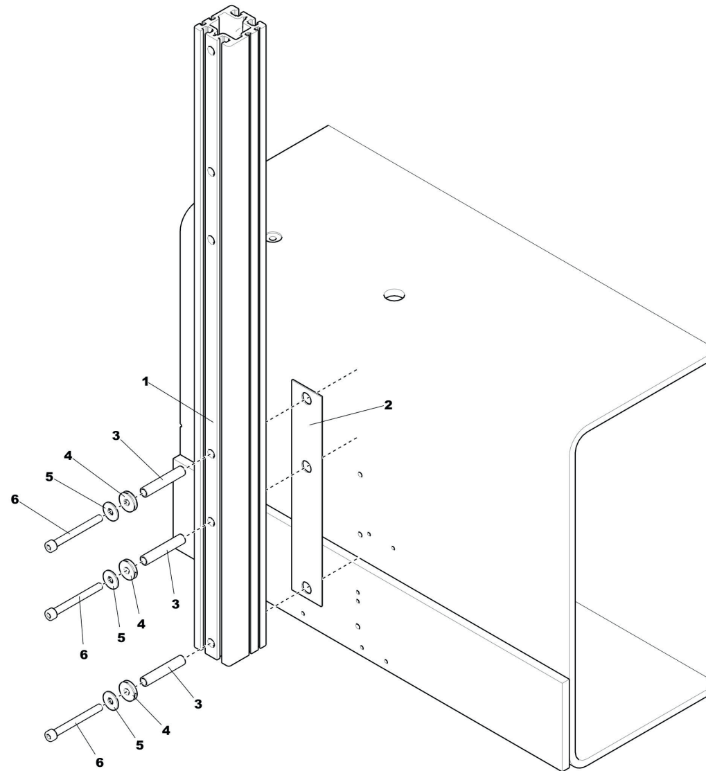
TDLE - 310 031 929 - Profilrohrbefestigung am Träger
