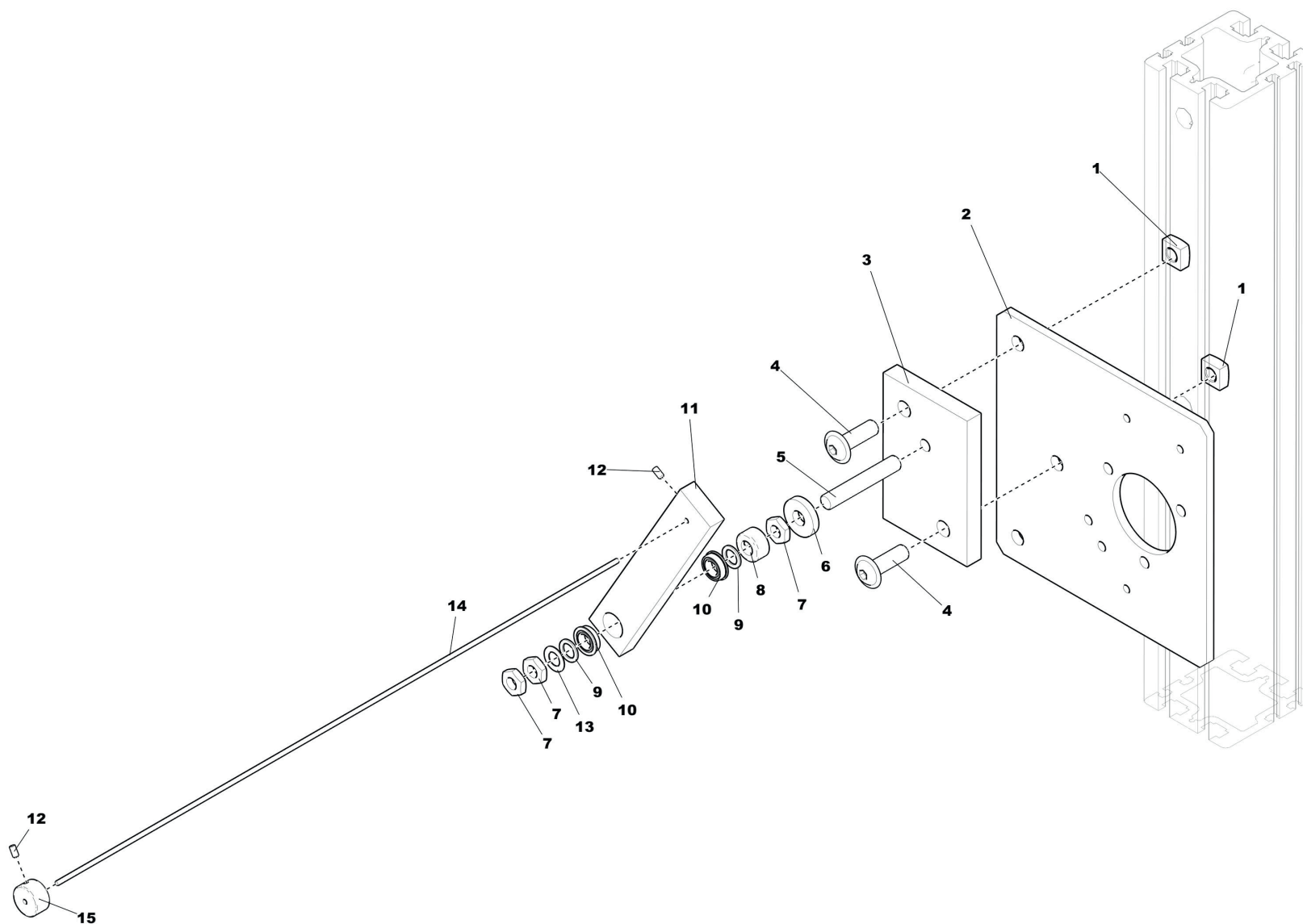
TDLE - 310 031 929 - Wippe/Abstreifer re
