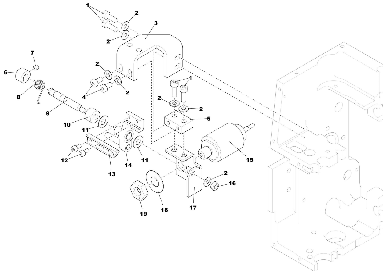
WKO-310 003 985 (B) - Nadelabschaltung / Needle Switching Off
