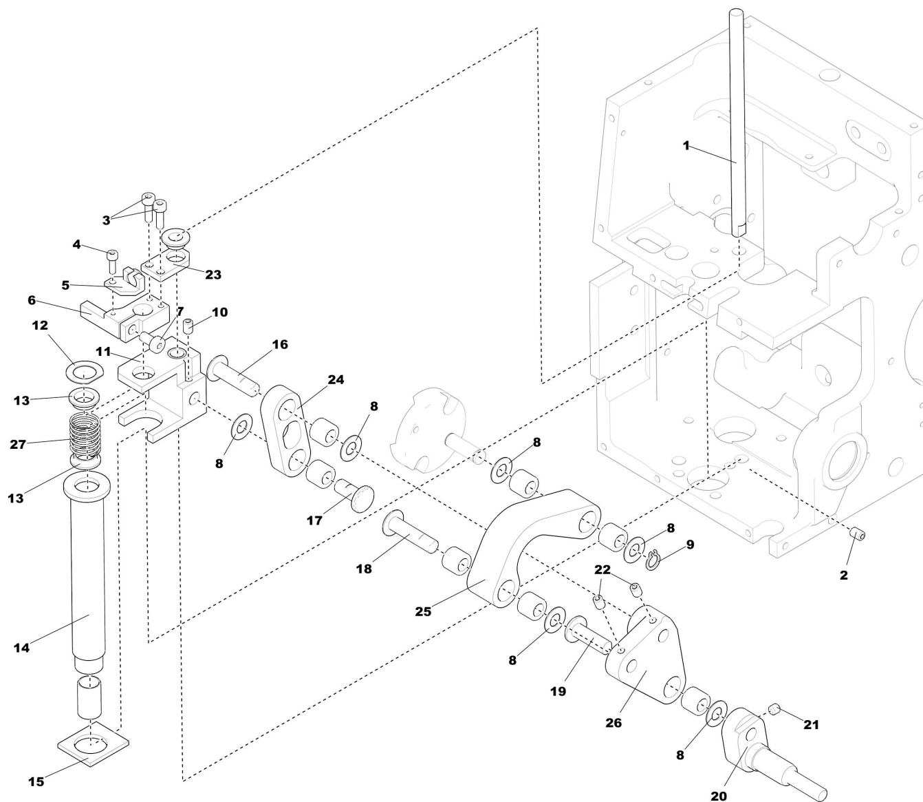
WKO-310 003 985 (B) - Stoffdrückerantrieb / Pressure Foot Drive
