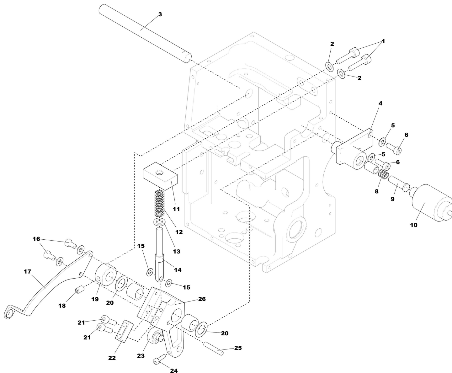
WKO-310 003 985 (B) - Fadengeber & Abschaltung W-Kopf/ Thread Take-up & Switch-off W-Head
