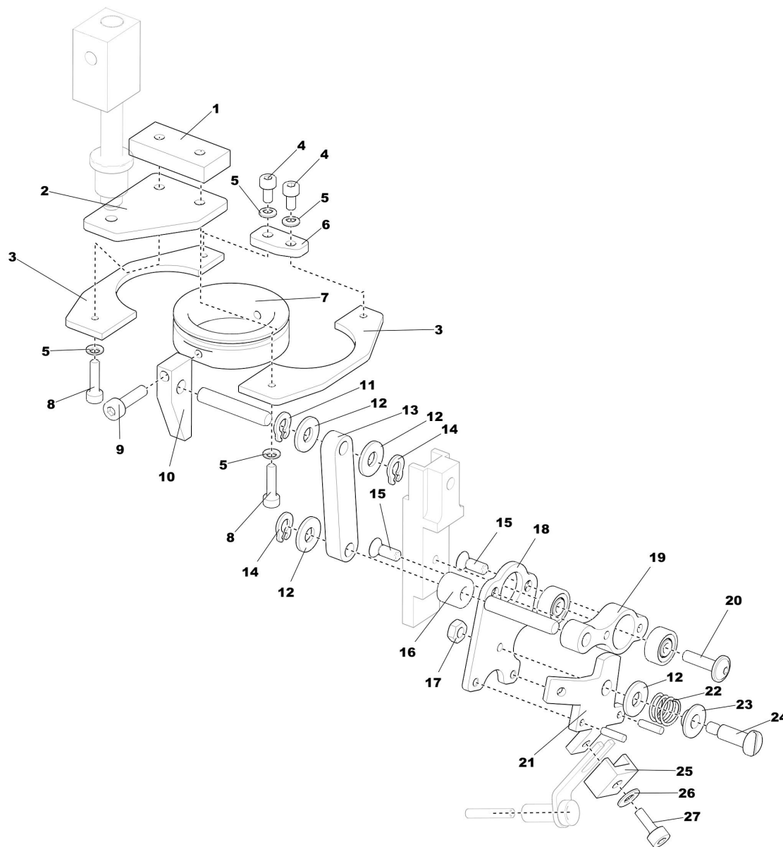
WKO-310 003 985 (B) - Zick-Zack W-Kopf / Zig-Zag W Head
