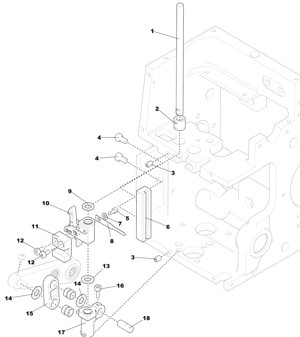
WKO-310 003 985 (B) - Springsticheinrichtung W-Kopf / Jump Stitch Device W Head
