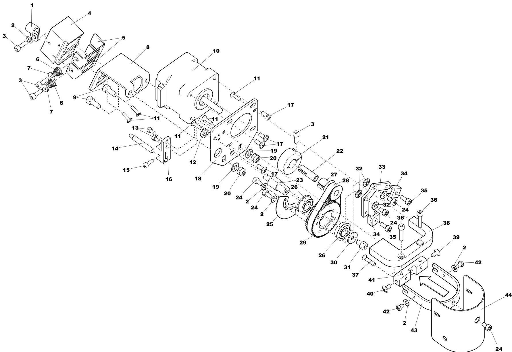
S36-37 - WKO-Auto. Wechselfuß -- Automatic Change Foot - 310 024 916 (B)
