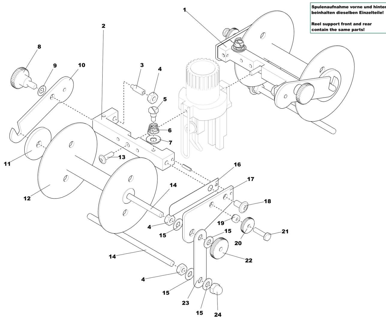
WKO-310 003 985 (B) - Spulenaufnahme / Reel support
