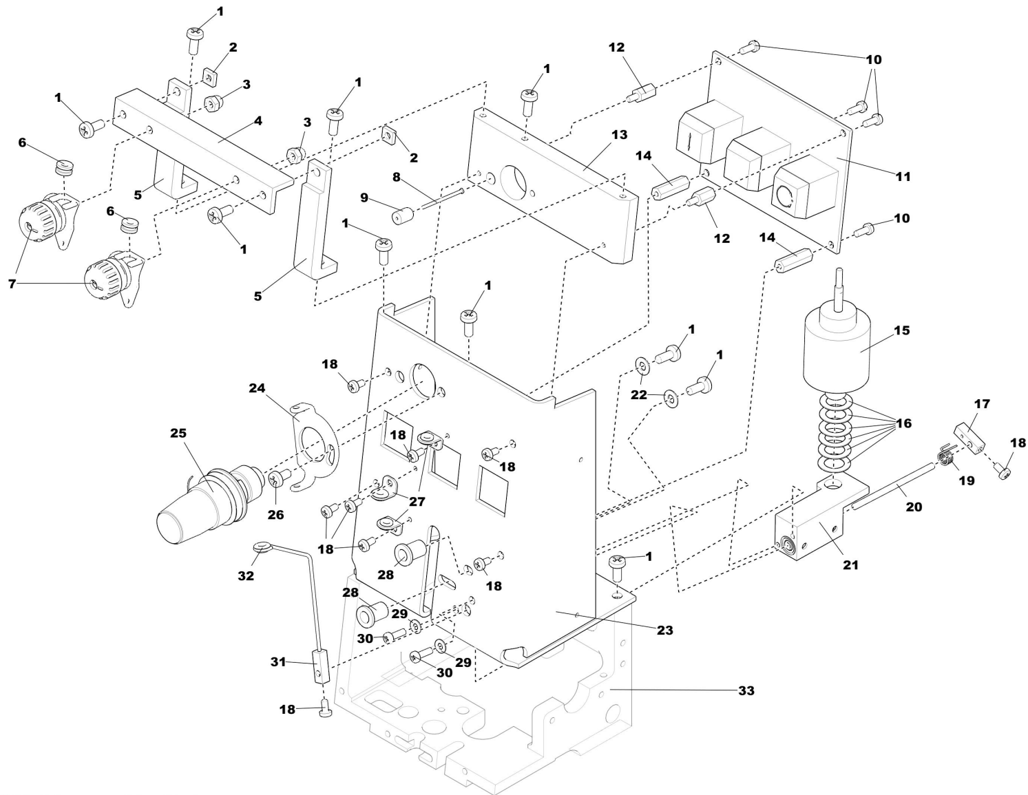
WKO-310 003 985 (B) - Fadenspannung / Thread Tension
