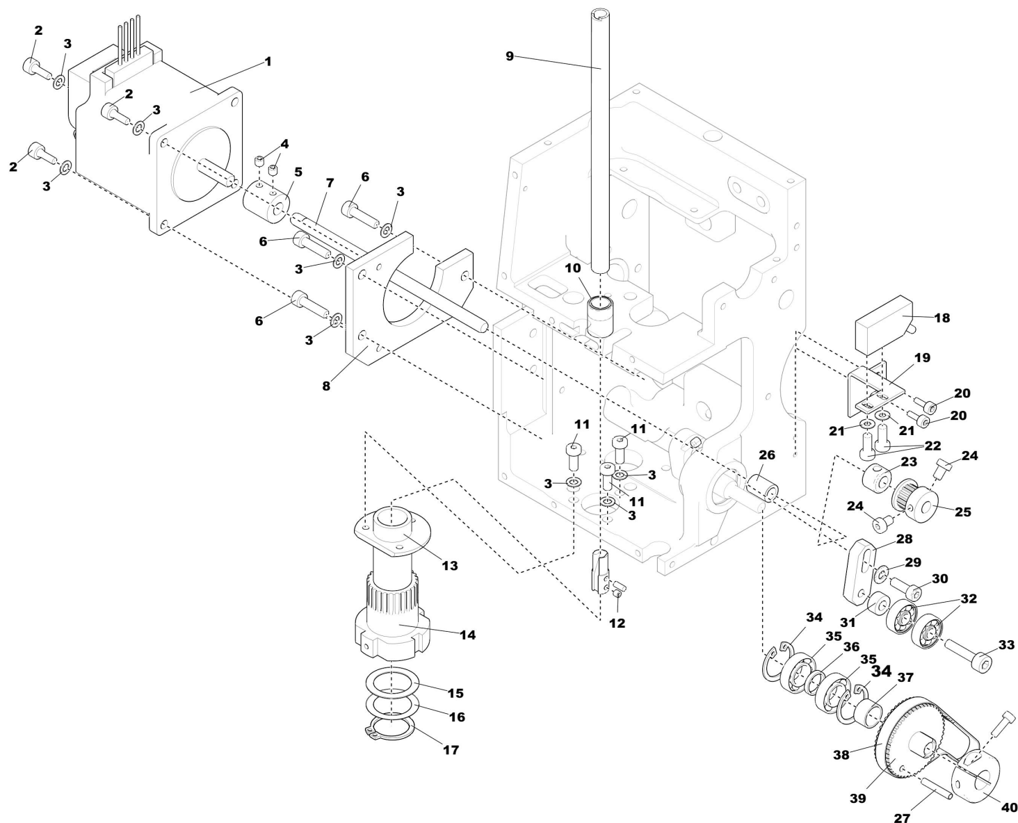
WKO-310 003 985 (B) - Stoffdrückerantrieb / Pressure Foot Drive
